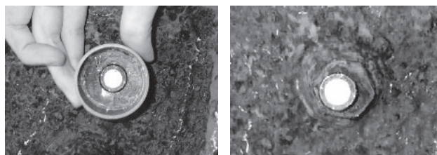
図-5 芯出し治具計測状況
