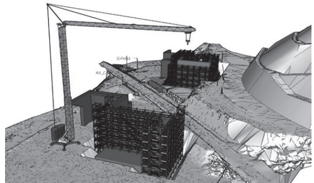
図-3 クレーン配置計画図
