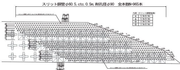
図-6 展開図 (右側1段目法面)
