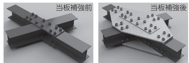
図-2 下横構部材交差部当板材の施工例
