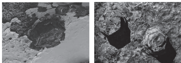
図-3 ボルト頭部腐食状況
